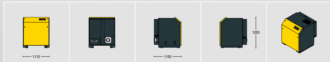
Серия СВ 166/236 С – с распределительным шкафом
