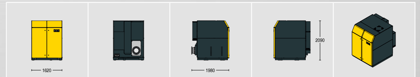
Серия ЕВ 441/791 С – с распределительным шкафом
